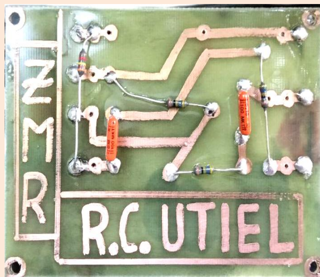
PLACA CIRCUITO IMPRESO DE LA INTERFACE
